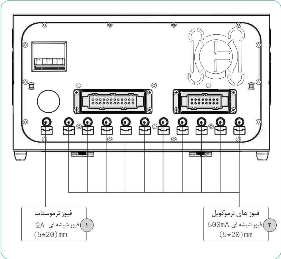
تصویر ۴: نمای پشت دستگاه ۹ زون و ۱۰ زون
