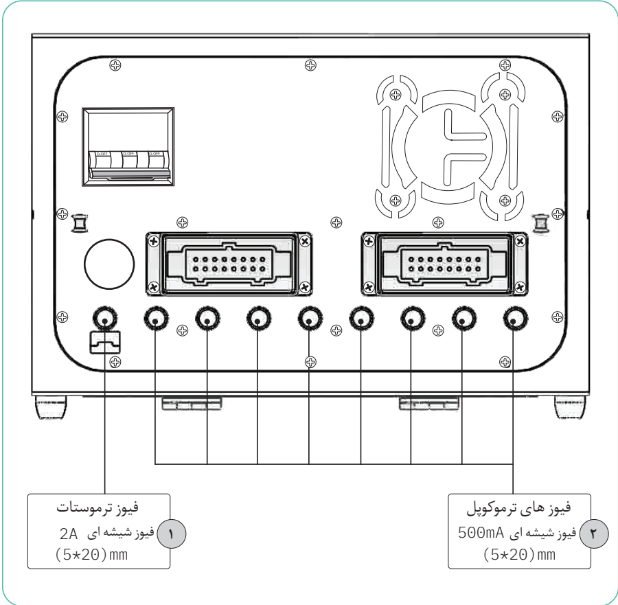
تصویر ۴: نمای پشت دستگاه ۸ زون
