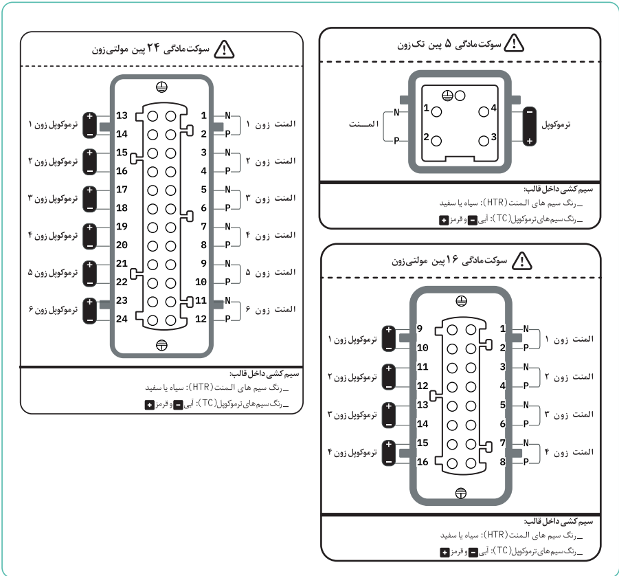
تصویر ۸: نقشه سوکت خروجی ۵، ۱۶، ۲۴
